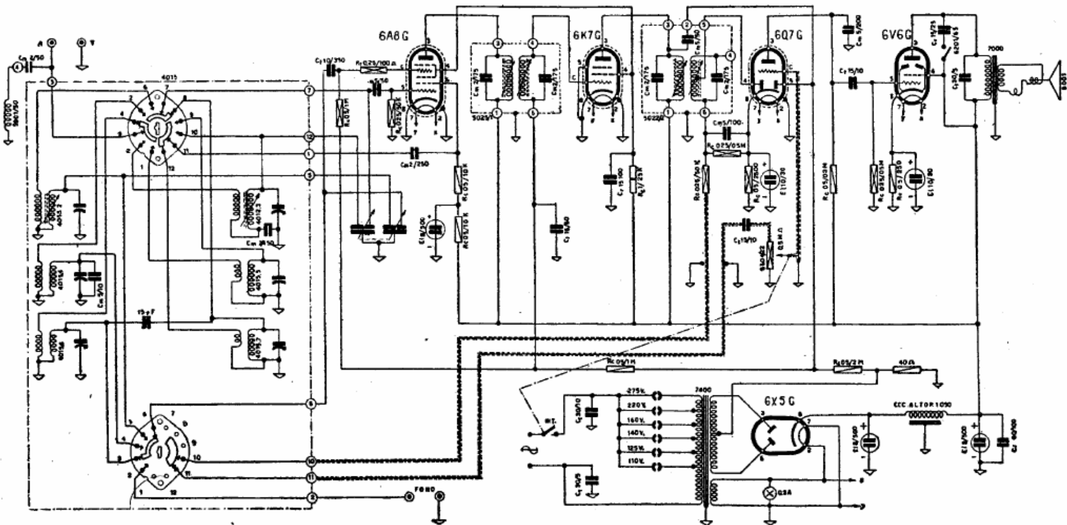
SIARE RADIO - Modelli 26 e 28 - Tre gamme d'onda. Media frequenza: 467 kc/s. Sensibilità: 40 microvolt. Potenza d'uscita: 4 watt circa. Consumo circa 60 watt. Produzione 1945-46.
